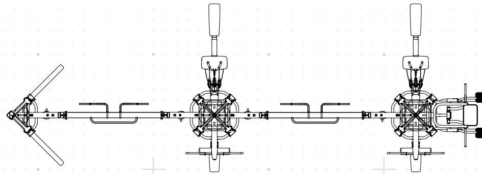
9站位 规格尺寸（长 x 宽 x 高） 388x1098x237厘米
