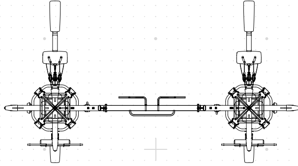
8站位 规格尺寸（长 x 宽 x 高） 388x685x237厘米
