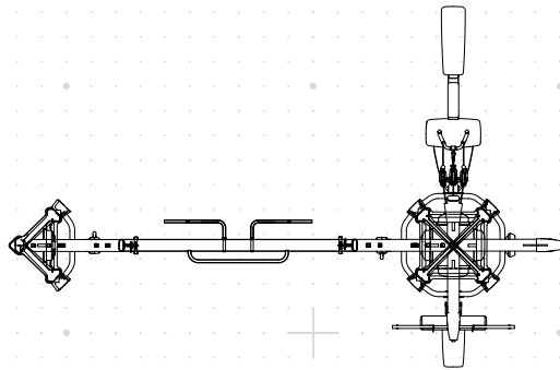
5站位 规格尺寸（长 x 宽 x 高） 388x601x237厘米
