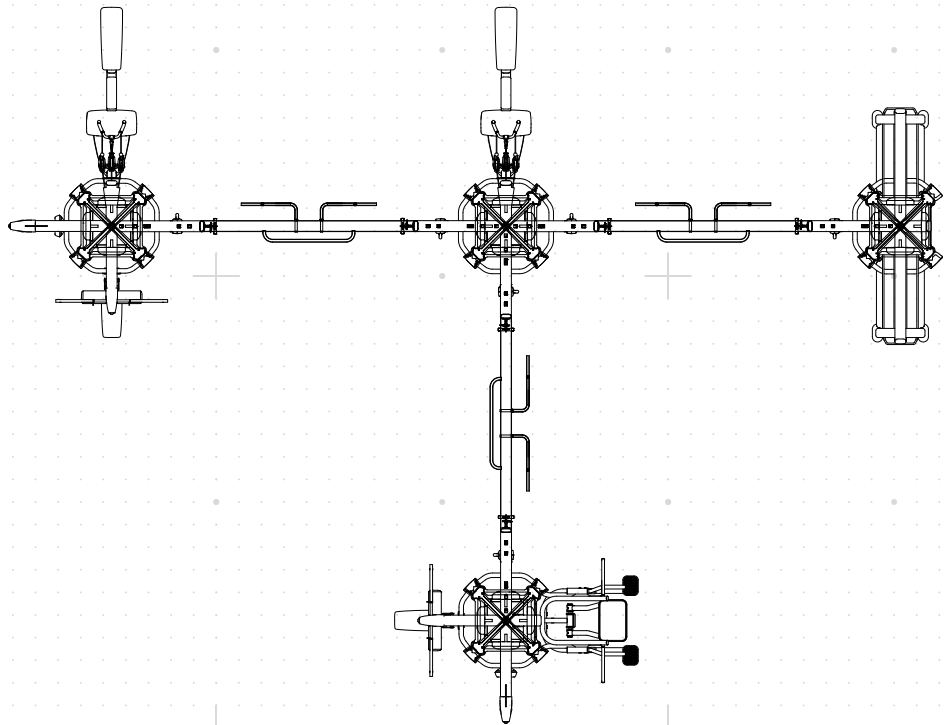
13站位（带储物空间） 规格尺寸（长 x 宽 x 高） 388x1097x237厘米
