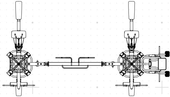
7站位 规格尺寸（长 x 宽 x 高） 388x703x237厘米
